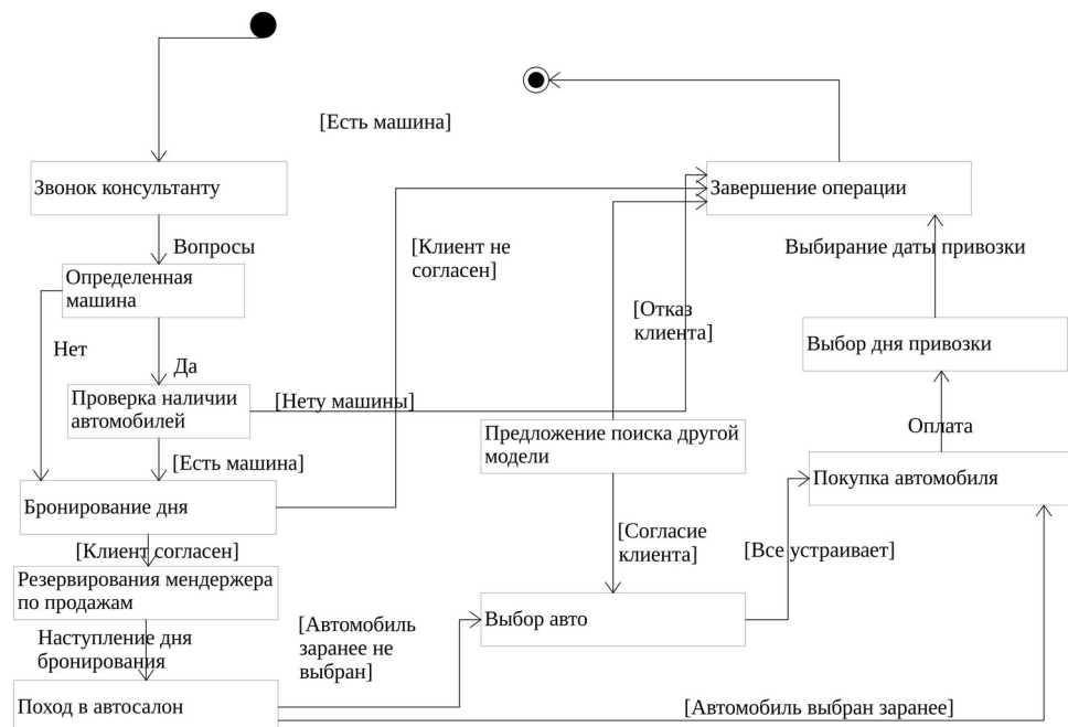
Рисунок 1 – Диаграмма состояний выбранной системы
